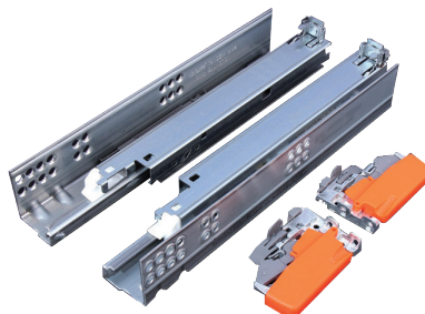
百隆缓冲托底轨
