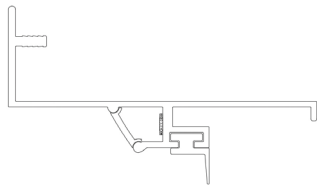
带灯顶护墙卡条
