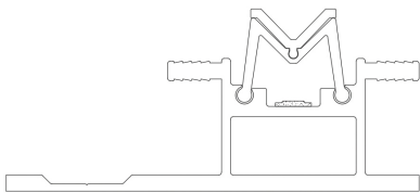
带灯护墙卡条
