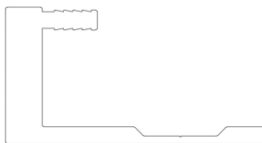
收口护墙卡条
